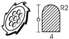
Hartmetallfräser Ø 110 x 4 mm, runde
