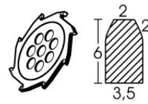
Hartmetallfräser Ø 110 x 3.5 mm
