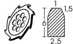
Hartmetallfräser Ø 110 x 2.5 mm
