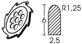
Hartmetallfräser Ø 110 x 2.5 mm, runde
